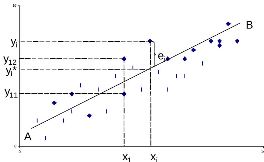
Figura 6. Diagrama de dispersión
